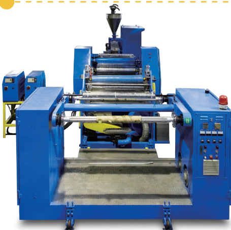
プラスチック製造ライン Plastic Sheet Production Line
